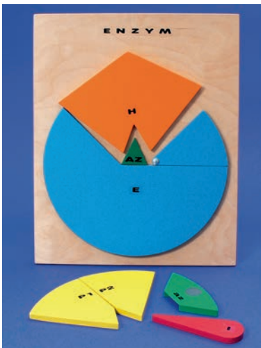
Schematisierte stark vergrößerte Darstellung eines komplexen Eiweißmoleküls
