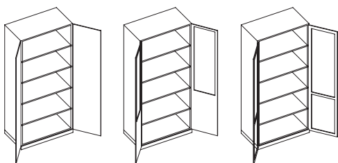
Schmale, 2-türige Ausführung, B x T x H: 900 x 550 x 2080 mm
