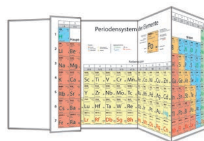
Schematische Darstellung der Faltung.
